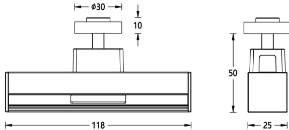
Wallwash
